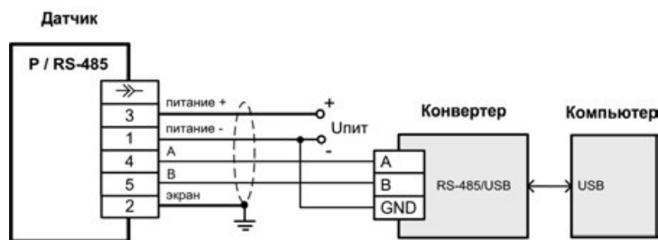
4-проводная линия (выходной сигнал – RS-485)
