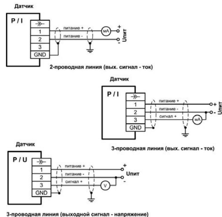
Рисунок 1 – Примеры схем подключения выходов для разъема DIN 43650A
